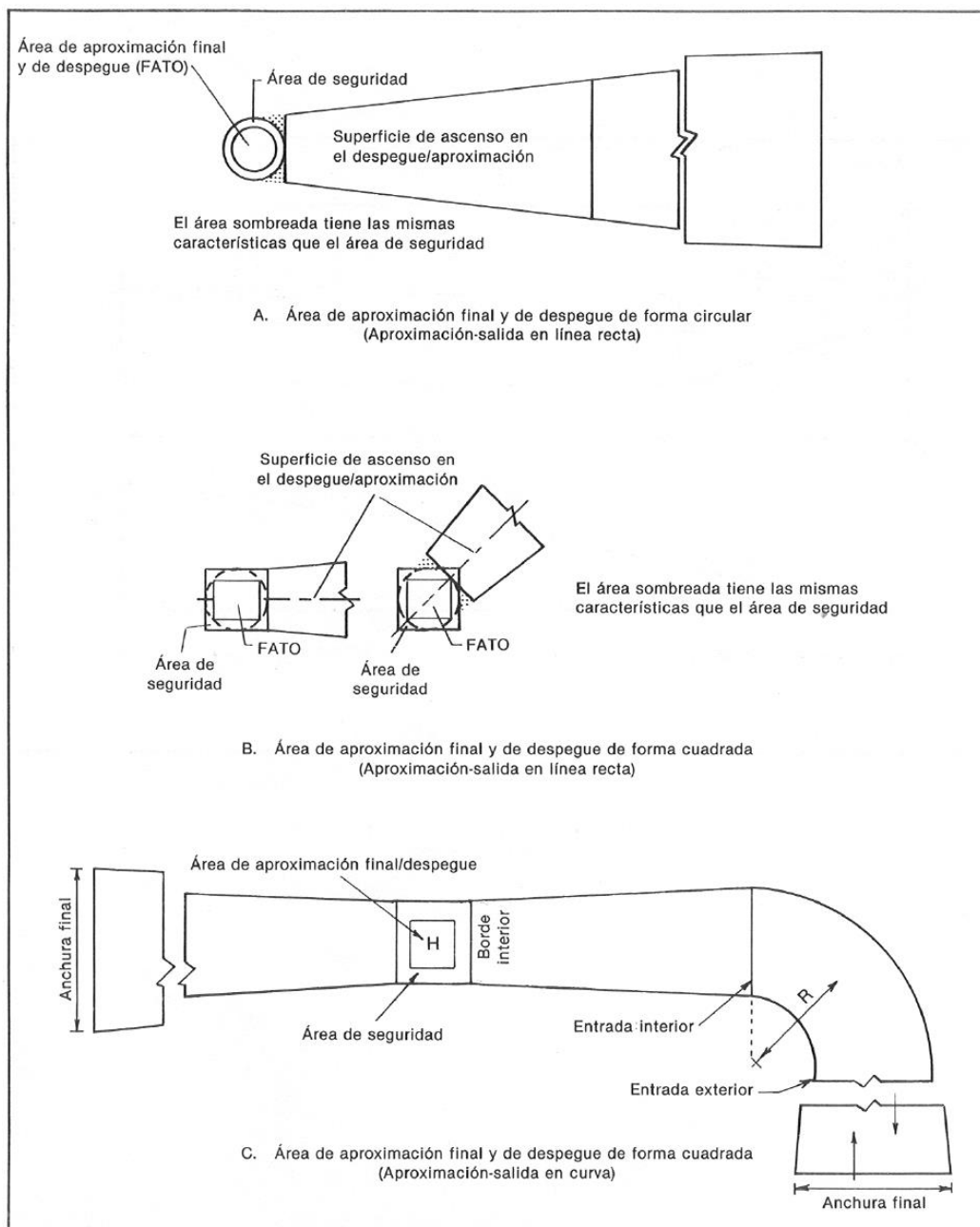
Figura 4-6H. Superficie de ascenso en el despegue/aproximación (FATO para vuelo visual)
