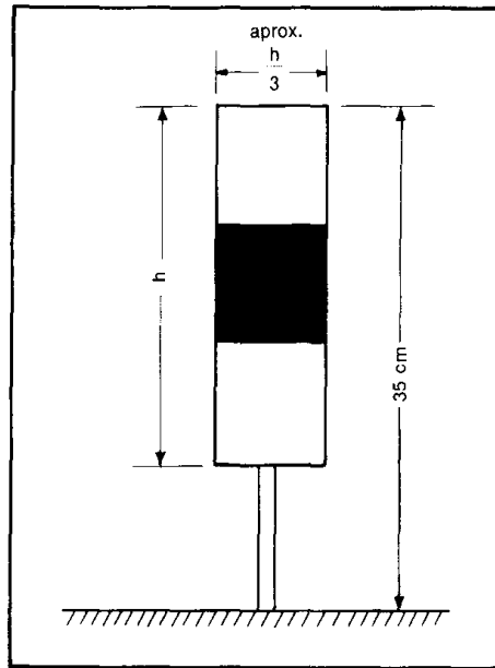
Figura 5-6H. Baliza de calle de rodaje aéreo
