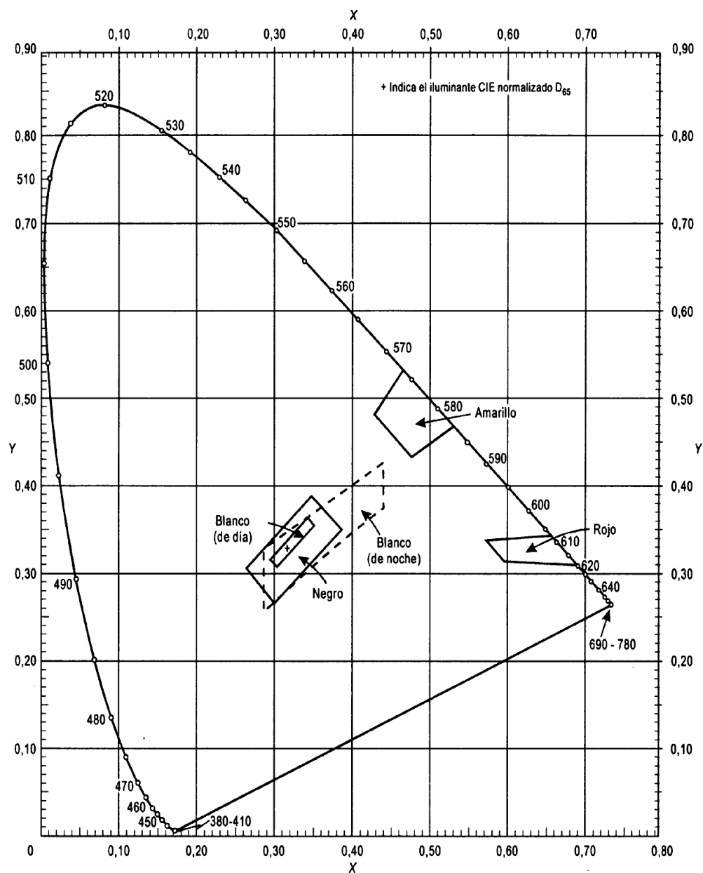
Figura A1 - 4. Colores de los letreos y paneles transiluminados ( Iluminación interna )
