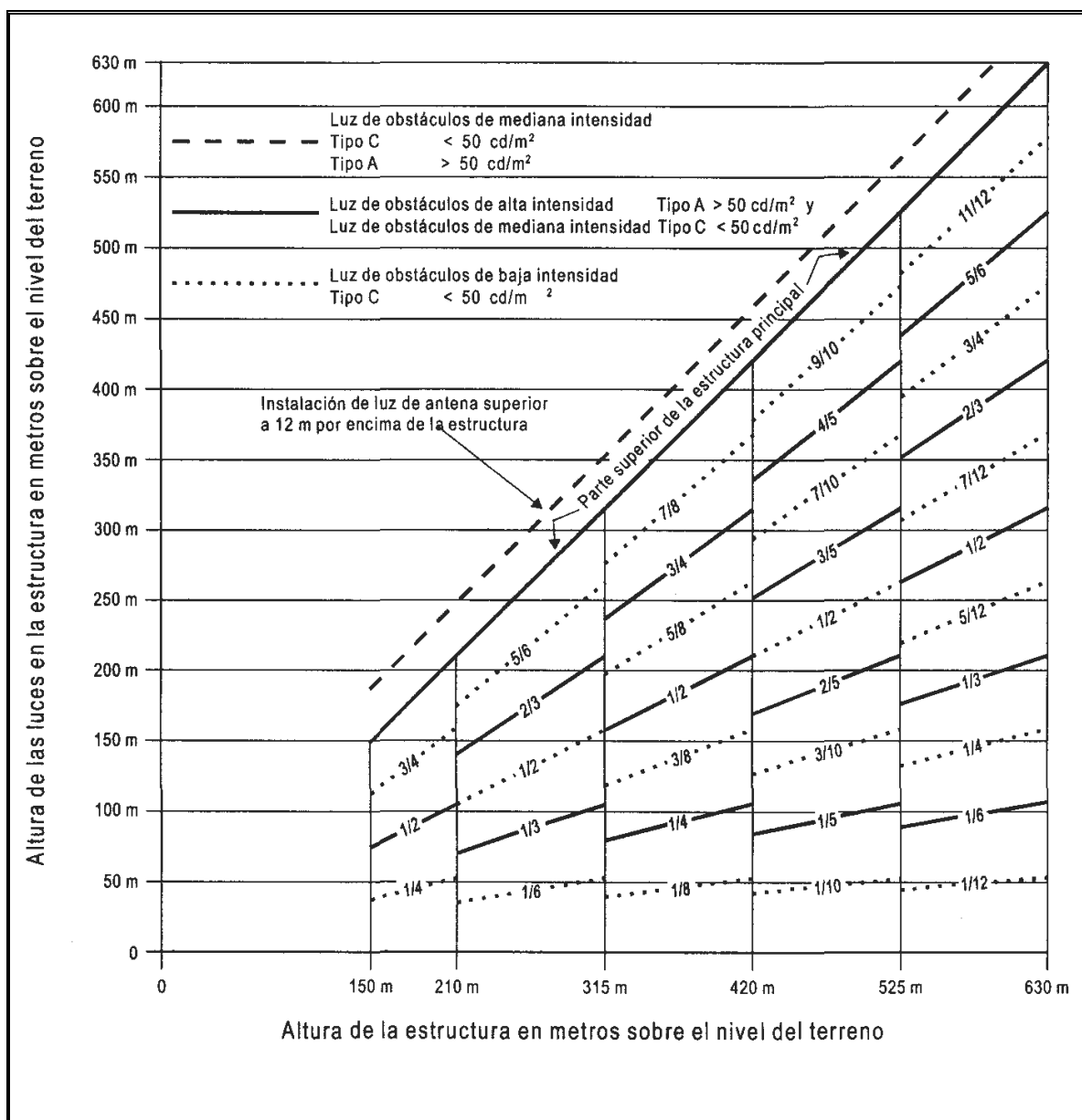
Figura A6 – 8. Sistema doble de iluminación de obstáculos de mediana / alta intensidad Tipo A / Tipo C.
