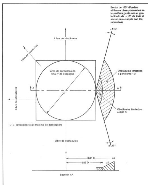
Figura 4-3H. Sectores limitadores de obstáculos en la heliplatforma. Helicópteros de rotor principal único y birrotores en paralelo
