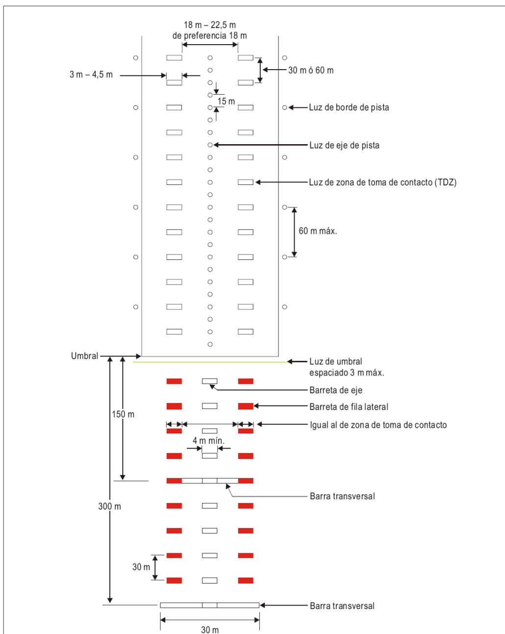
Figura 5-13. Iluminación de pista y de los 300m internos de la aproximación, en las pistas para aproximaciones de precisión de precisión de Categoría II y III
