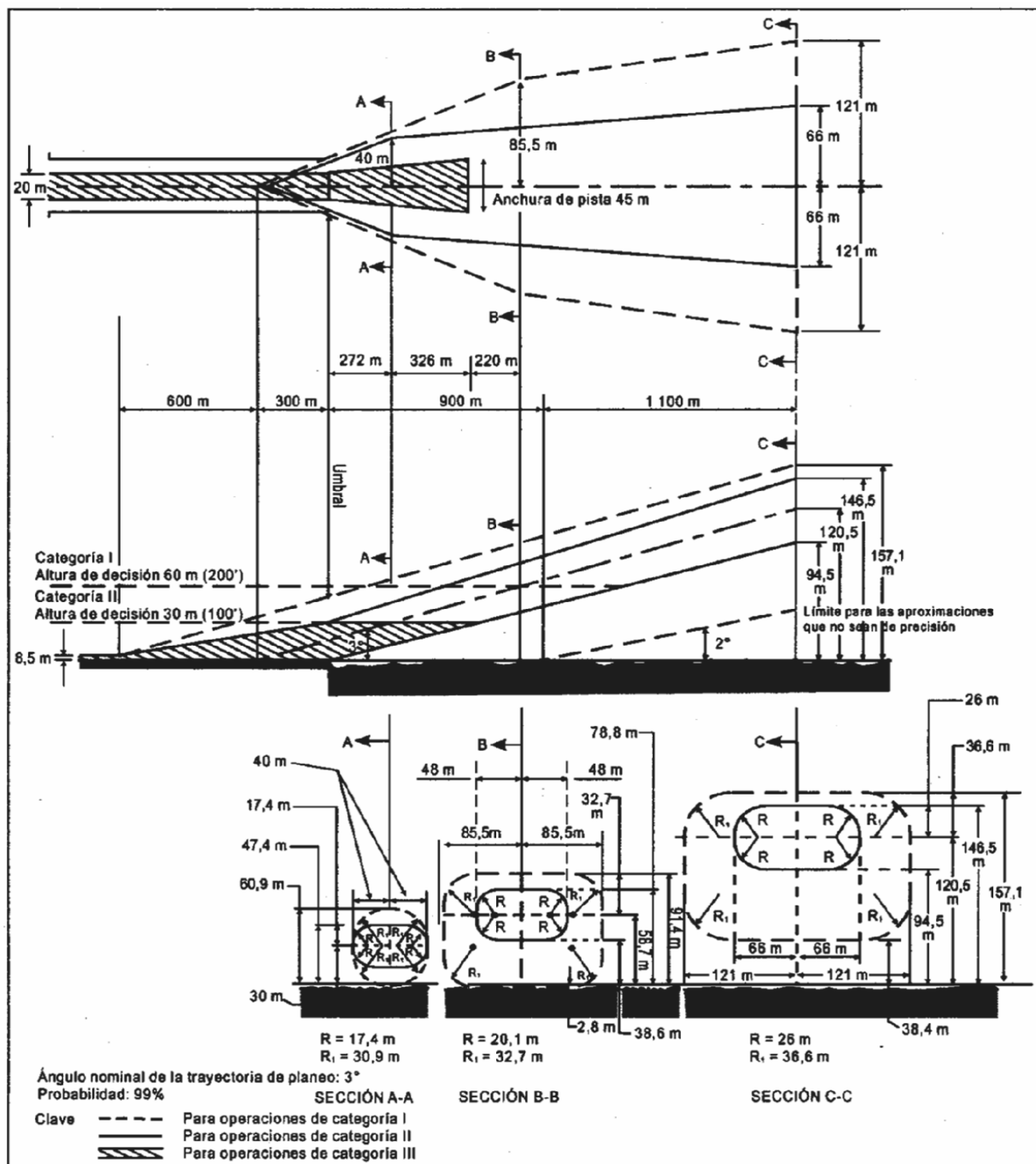
Figura A – 3. Parte nivelada de la franja de una pista para aproximaciones de precisión cuyo número de clave sea 3 ó 4.
