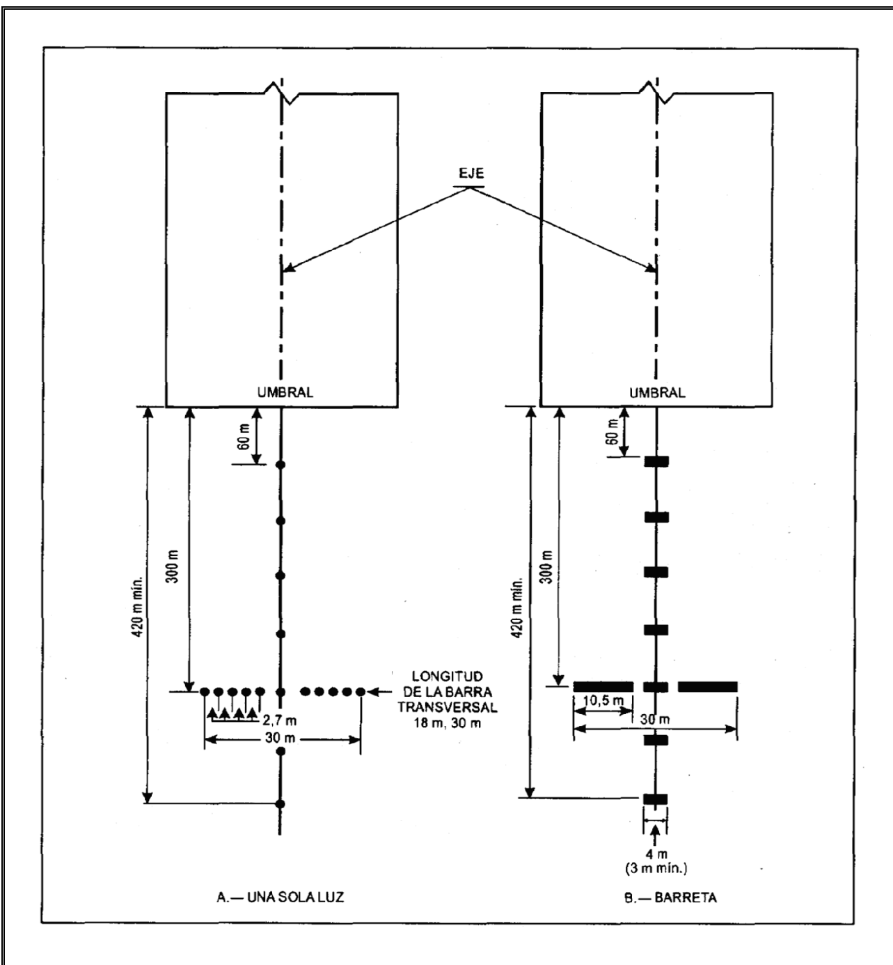
Figura A – 5. Sistemas sencillos de iluminación de aproximación.
