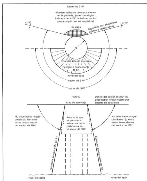
Figura 4-2H. Sector libre de obstáculos de la heliplatforma
