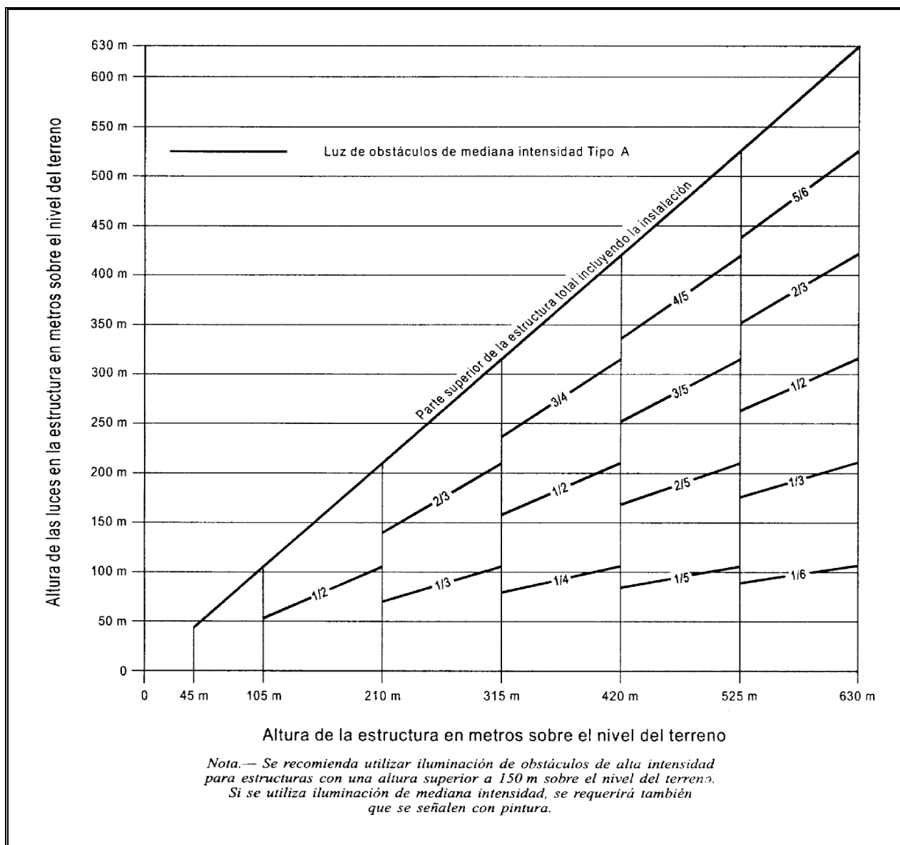
Figura A6 - 1. Sistema de iluminación de obstáculos con luces blancas de destello de mediana intensidad Tipo A
