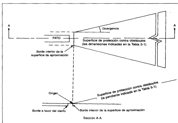
Figura 5-13H. Superficie de protección contra obstáculos para sistemas visuales indicadores de pendiente de aproximación
