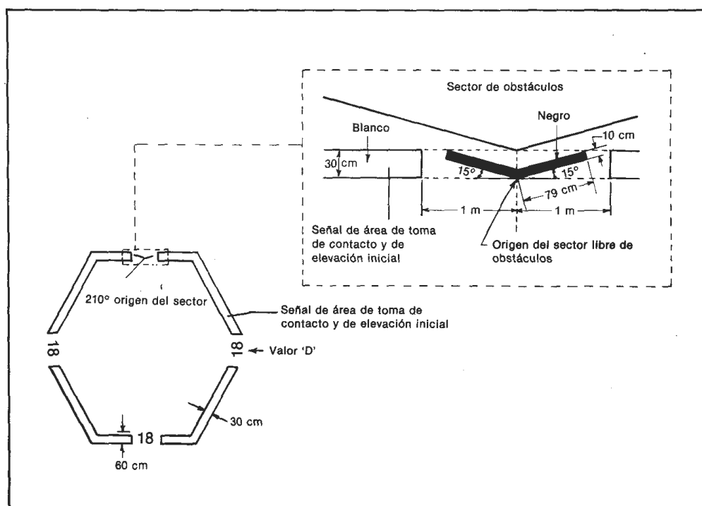
Figura 5-5H. Señal de sector despejado de obstáculos de heliplateaforma
